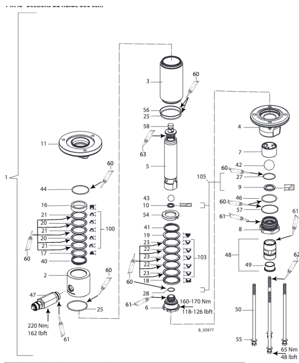
Sections du fluide 600 ccm
