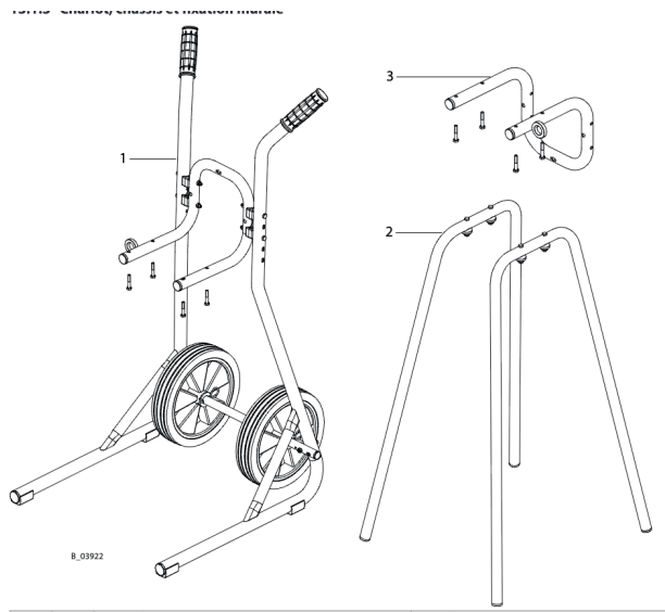
Chariot, châssis et fixation murale
