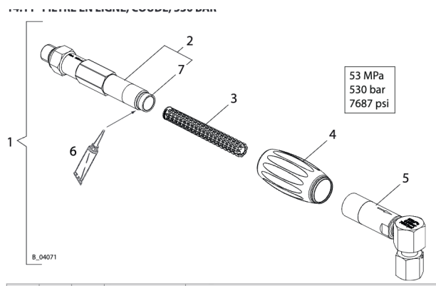
FILTRE EN LIGNE, COUDÉ, 530 BAR
