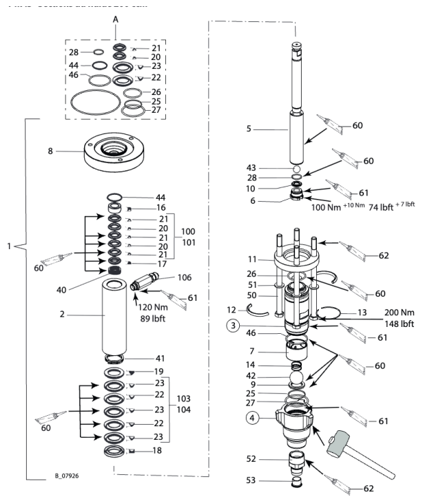
Sections du fluide 200 ccm
