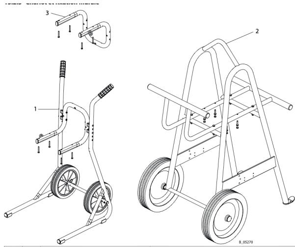
Chariot et fixation murale
