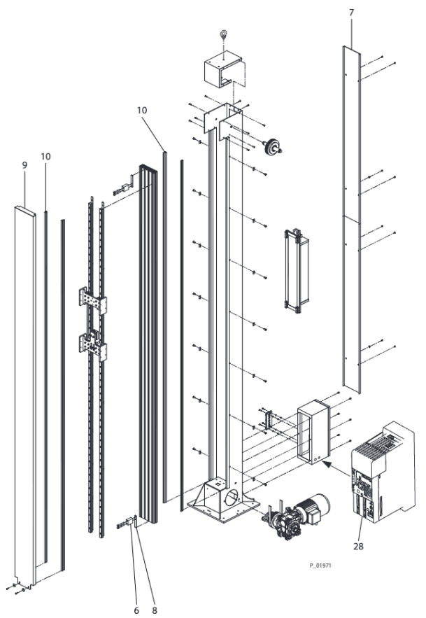
BÂTI DE LEVAGE VU1
