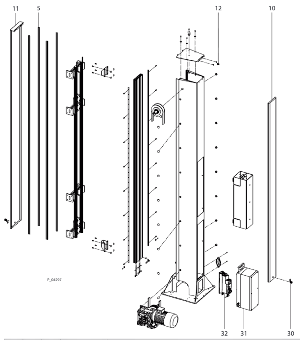
BÂTI DE LEVAGE VU3
