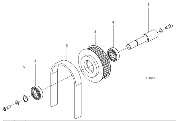
UNITÉ DE RENVOI VU3
