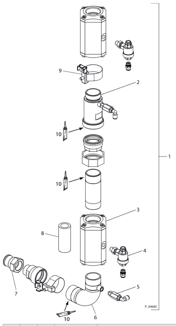
POMPE PÉRISTALTIQUE PP25S, DROITE
