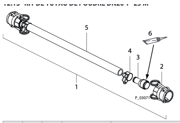
KIT DE TUYAU DE POUDRE DN20 1 " 25 M
