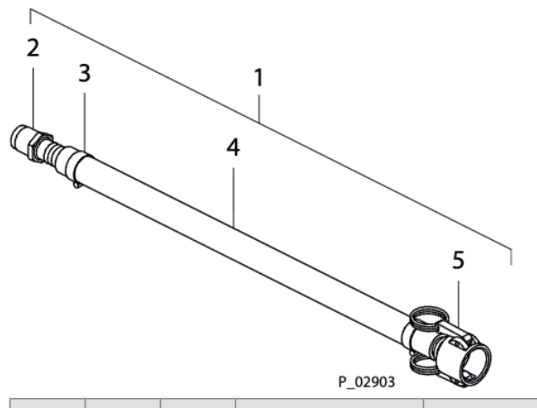
KIT DE TUYAU DE POUDRE DN20
