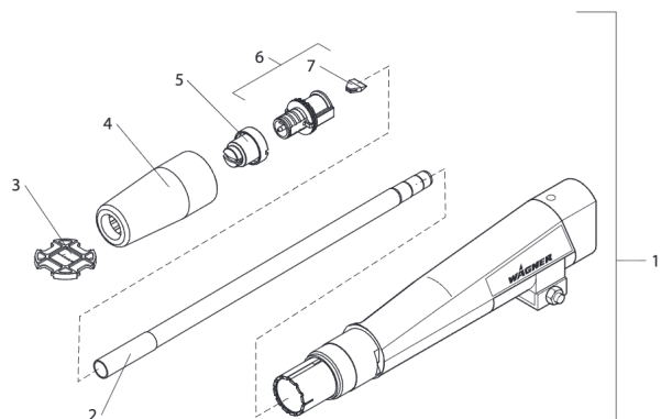
PISTOLET AUTOMATIQUE CORONA PEA-C4 HICOAT
