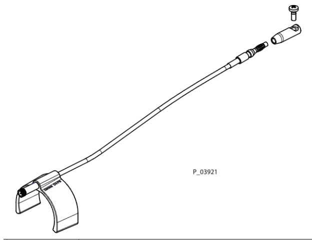
KIT DE POST-ÉQUIPEMENT CORONASTAR PEA-C4 F5
