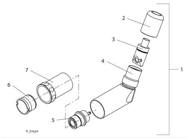
ADAPTATEUR COUDÉ WA60 C4
