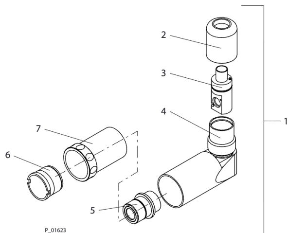
ADAPTATEUR COUDÉ WA90 C4
