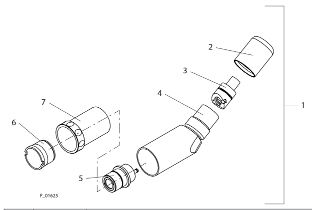
ADAPTATEUR COUDÉ WA30 C4
