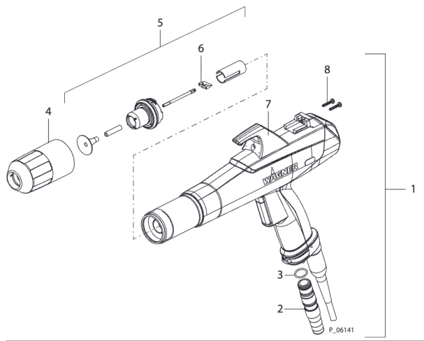
PISTOLET MANUEL ÉMAIL PEM-X1E AVEC BUSE À JET ROND
