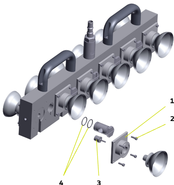
Ensemble support 12 bols tous diamètres (80 mm inclus) pour THV, T8 et T8X
