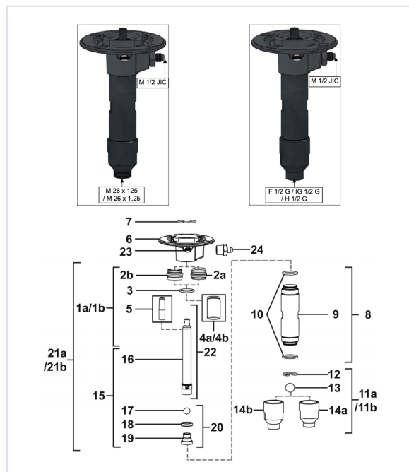
Vue éclatée extraite de la nomenclature SAMES doc. 582110110
