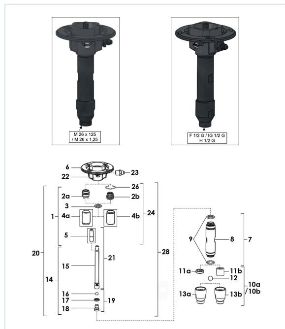
Vue éclatée extraite de la nomenclature SAMES doc. 582019110
