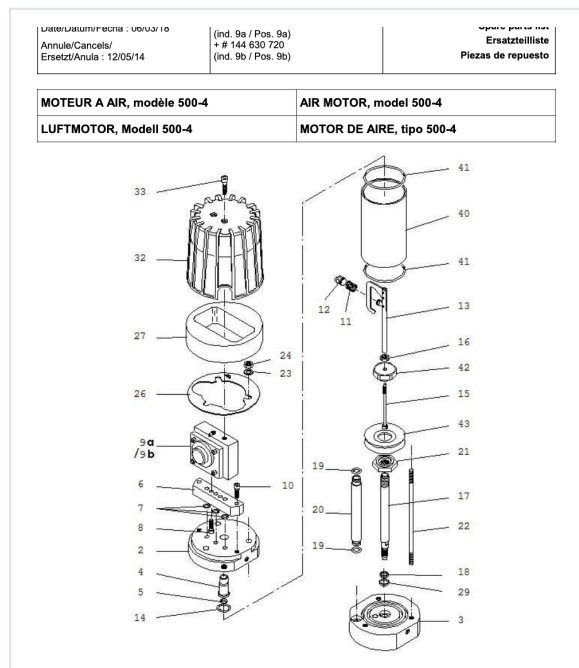
Vue éclatée extraite de la nomenclature SAMES doc. 582016110
