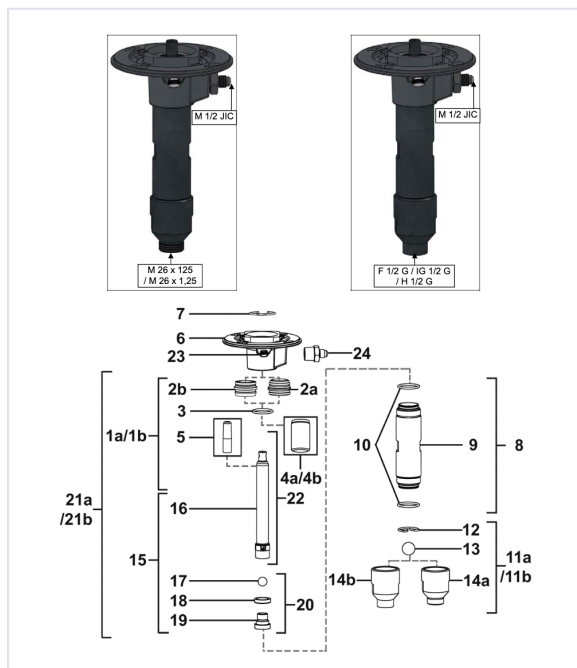
Vue éclatée extraite de la nomenclature SAMES doc. 582093110
