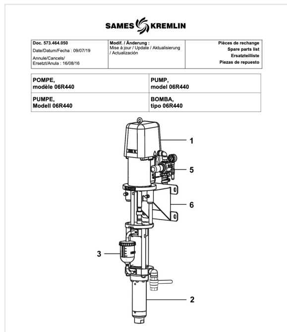
Vue éclatée extraite de la nomenclature SAMES doc. 582053110
