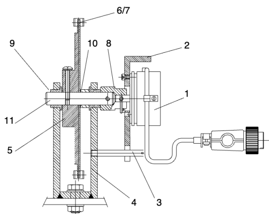
Montage du potentiomètre
