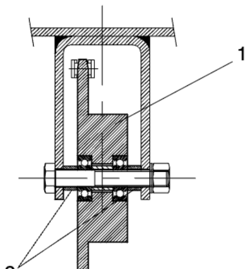
Montage de la roue dentée folle (haut)
