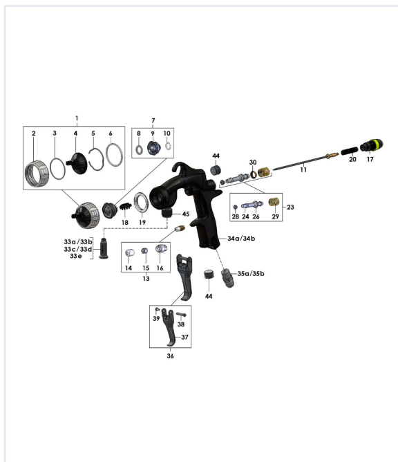
Vue éclatée extraite de la nomenclature SAMES doc. 582097110
